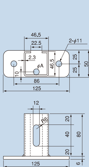
MHG-80 寸法図
