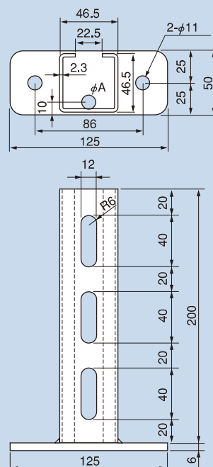
MHG-200 寸法図
